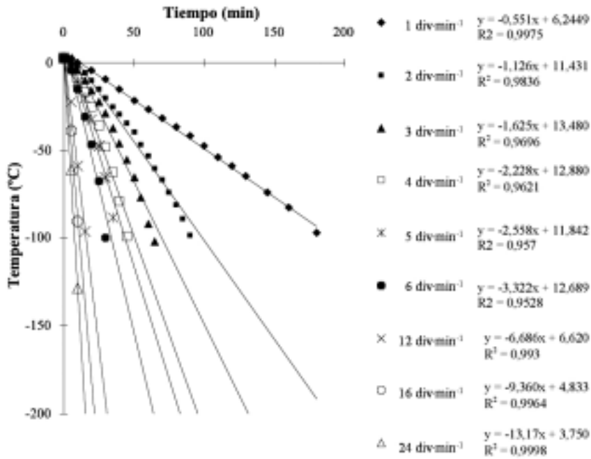
Figura 2. Líneas de mejor ajuste para diferentes tasas de descenso (div·min -1 ) de la placa porta-muestras obtenidas con del equipo mecánico de congelación, entre 3,5 y -100°C. A la derecha se indican las ecuaciones de cada una de las rectas obtenidas. La pendiente de cada recta indica la tasa de congelamiento (°C·min -1 ) obtenida para cada velocidad utilizada.
